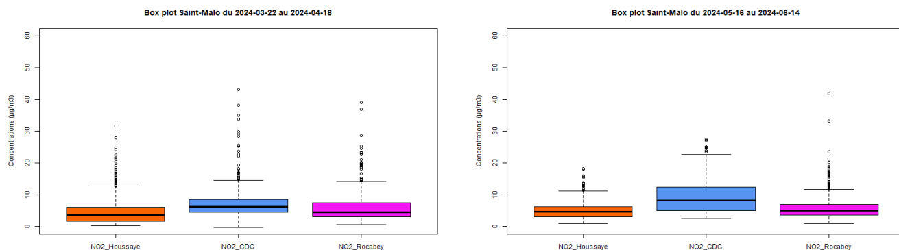
Figure 17 : Box plot des concentrations en NO 2 mesurées sur les deux campagnes (données horaires)
