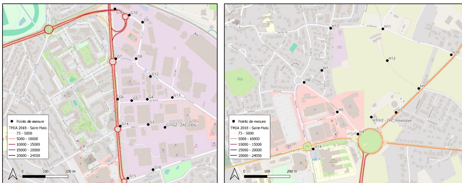
Figure 12 : Carte du TMJA (2018) sur les 2 zones d'étude (gauche : ZAC CDG ; droite : ZAC de la Houssaye)
