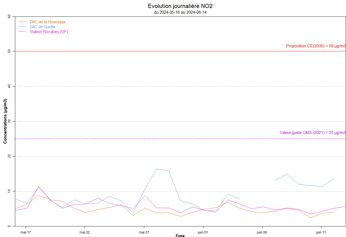
Figure 19 : Evolution journalière des concentrations en NO 2 lors de la campagne estivale (µg/m 3 )
